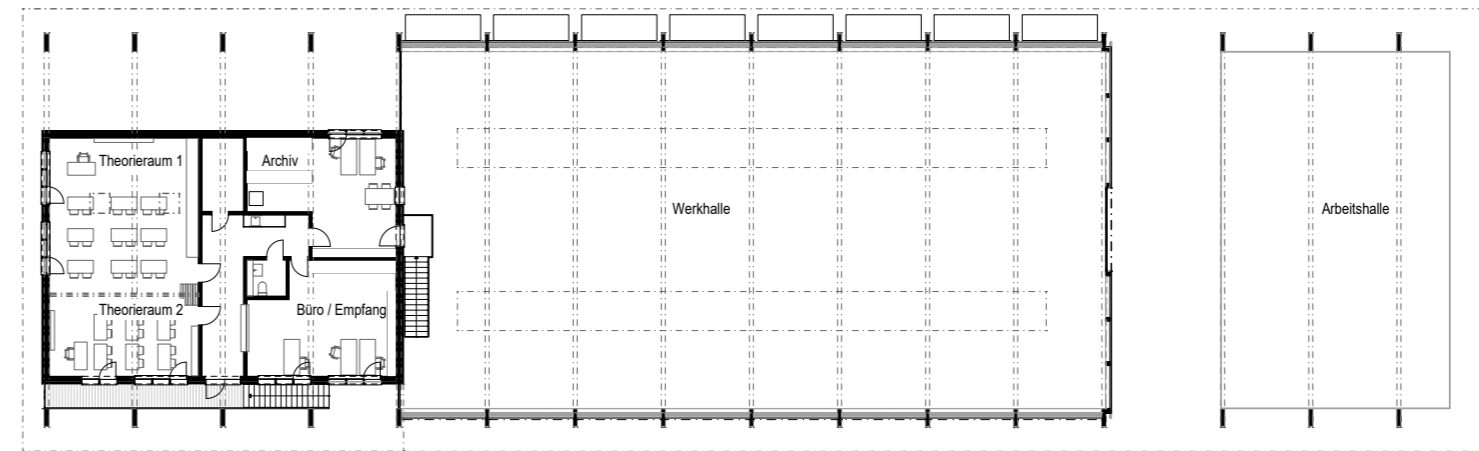
Grundriss OG
