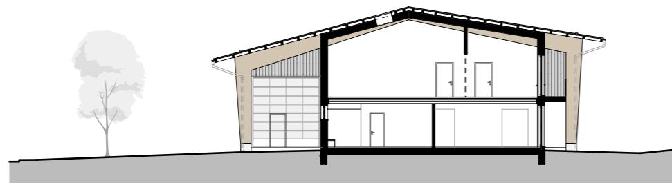
Schnitt Schulungsgebäude
