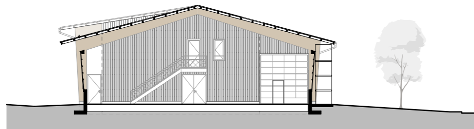
Schnitt Werkhalle Mst. 1:300
