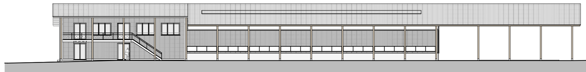
Südost Fassade
